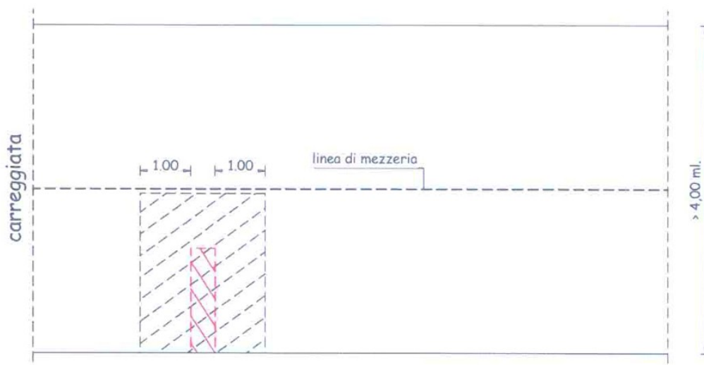
figura 8 - scavo trasversale alla carreggiata
