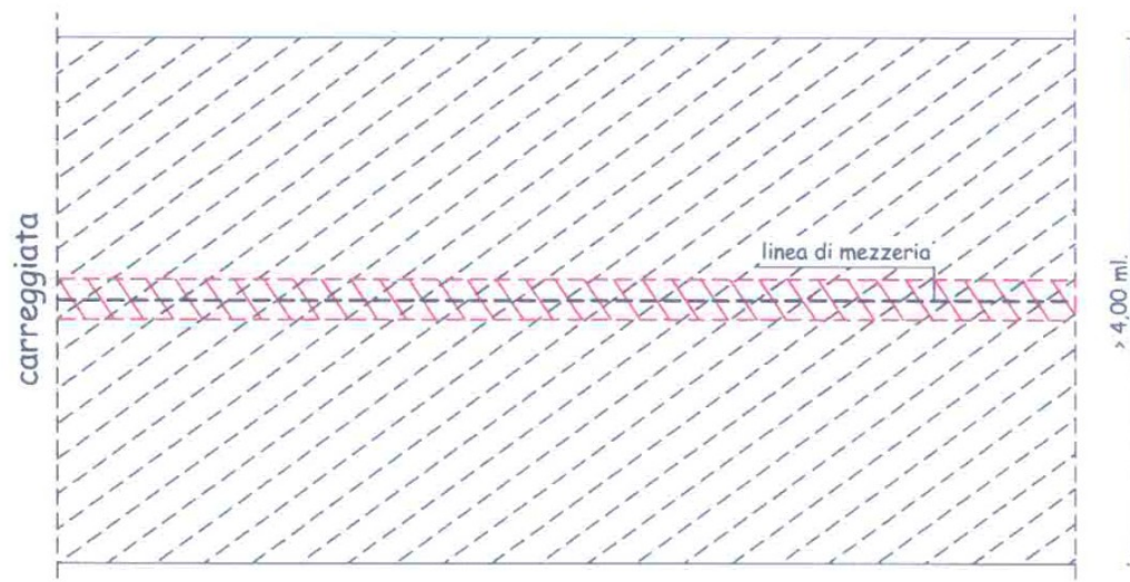
figura 14 - scavo al centro della strada
