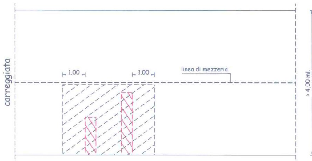
figura 10 - doppio scavo trasversale alla carreggiata
