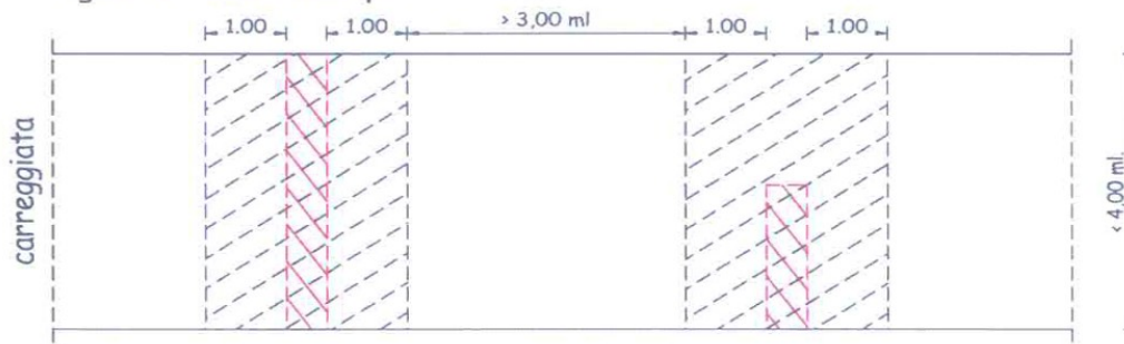
figura 6 - scavi multipli
