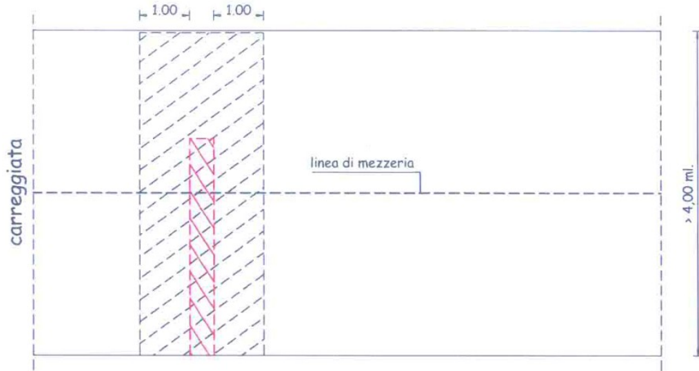
figura 9 - scavo trasversale alla carreggiata
