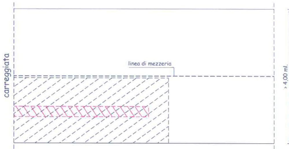
figura 7 - scavo longitudinale alla carreggiata
