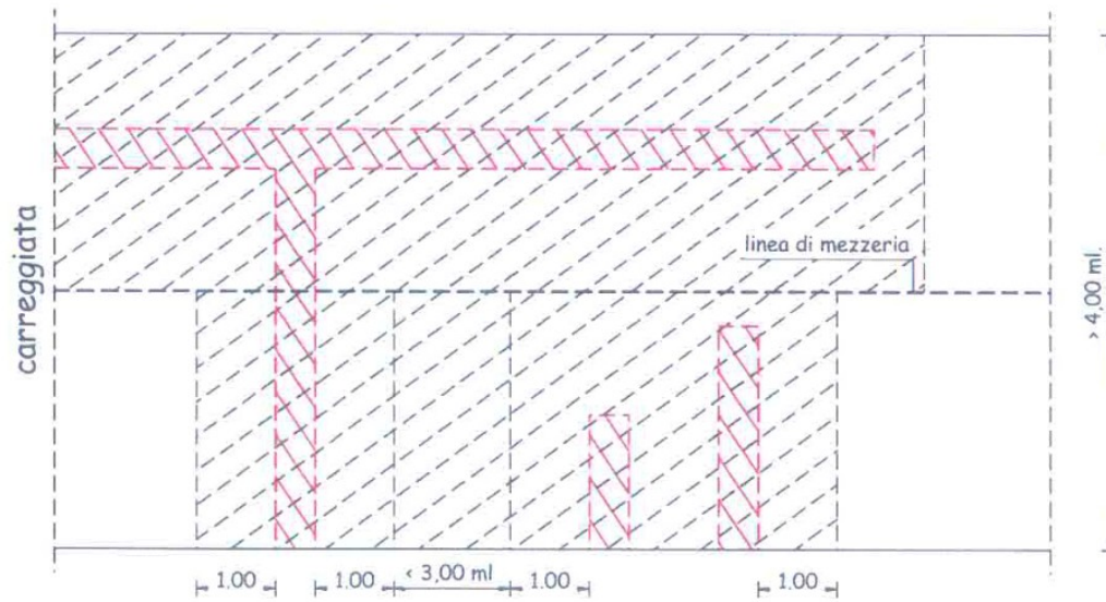
figura 12 - scavi multipli
