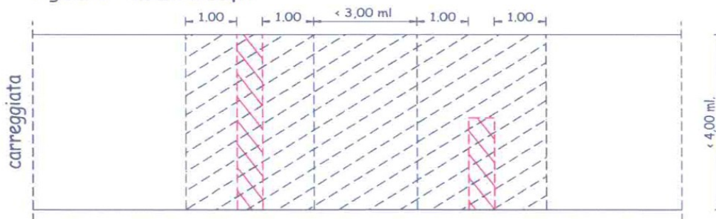
figura 5 - scavi multipli
