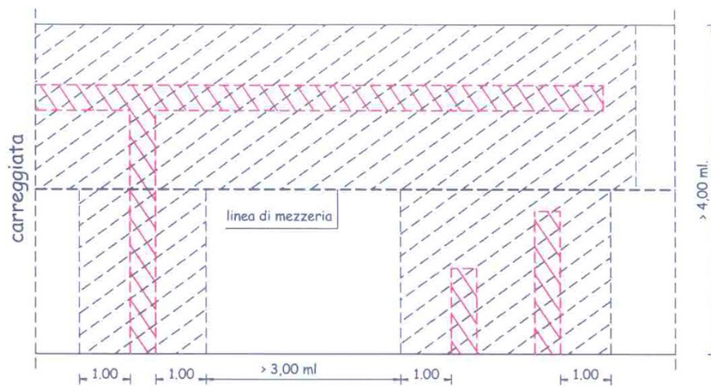
figura 13 - scavi multipli
