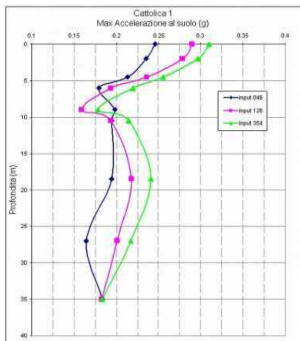
Figura 5.17 – Distribuzione delle accelerazioni orizzontali di picco per i tre input sismici di riferimento (modello "Cattolica 1").
