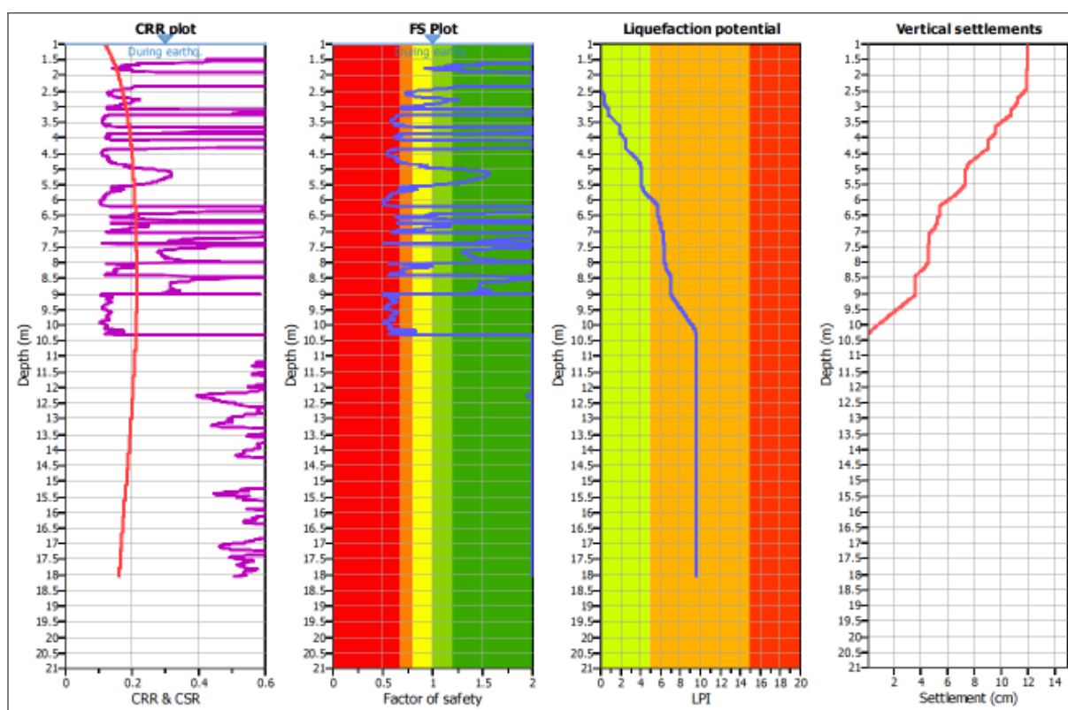
Figura 5.28 - Plottaggio delle verifiche di liquefacibilità e cedimenti relativi alla prova penetrometrica P1CPTE1
