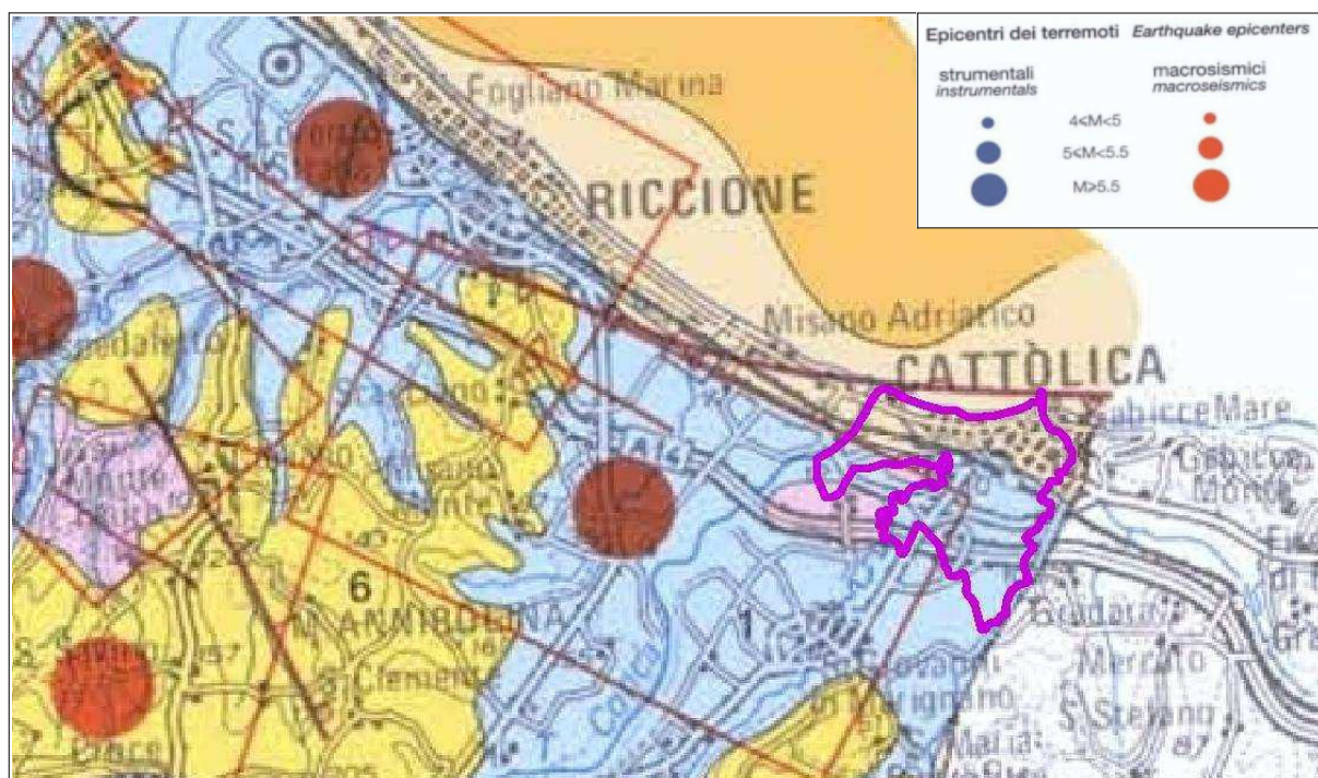
Figura 5.1– Sovrapposizione del territorio comunale di Cattolica con la Carta Sismotettonica della Regione Emilia-Romagna (2004). Si riporta uno stralcio della legenda relativamente alla classificazione degli ipocentri dei terremoti strumentali di M_w > 4 e l'epicentro dei più significativi effetti macrosismici. La fonte regionale degli eventi sismici riportati è il catalogo parametrico nazionale dei terremoti storici (CPTI, 1999).
