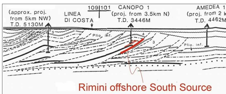
Figura 5.7 – La sorgente "Rimini offshore south" proiettata sulla Sezione Amedea-Mte. Amiata (da Bally et al., 1986).
