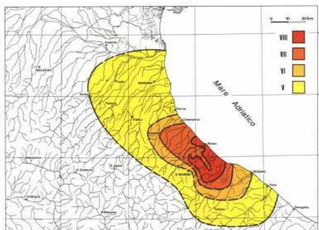
Figura 5.6 – Carta delle isosisme dell'evento del 25 dicembre 1786. Si noti la caratteristica propagazione degli effetti in prevalente direzione parallela alla costa (da Ferrari, 1986).
