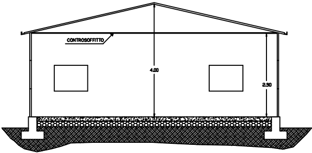
SEZIONE A-A
