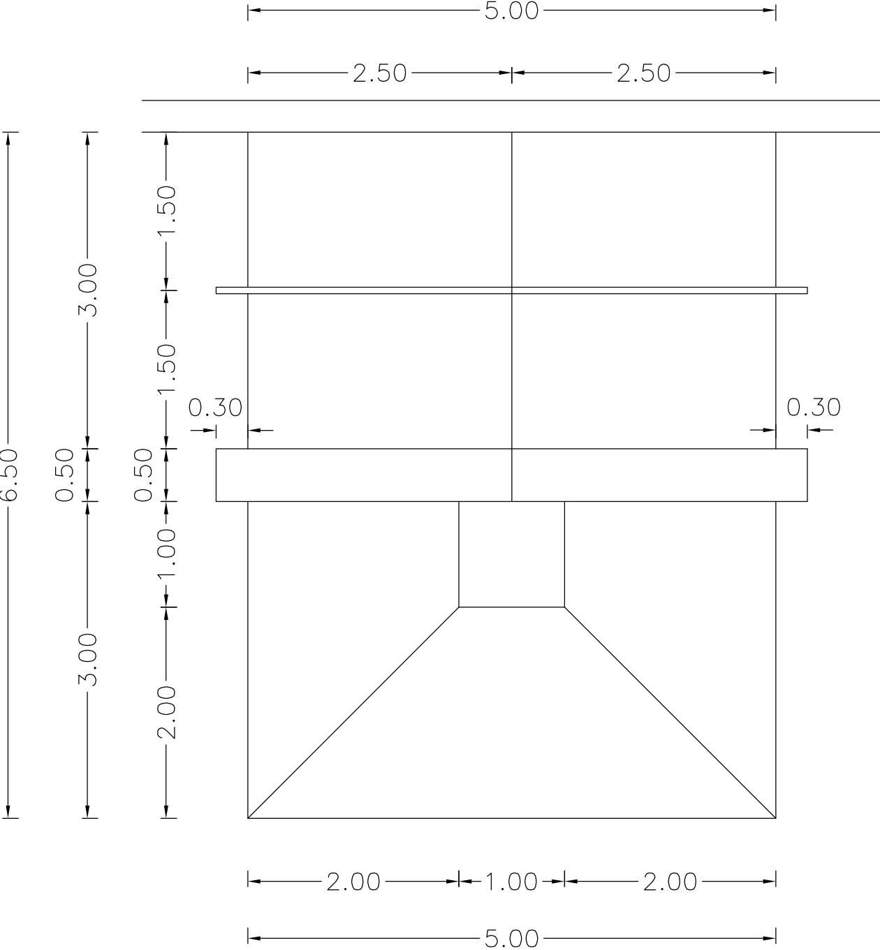
PIANTA
