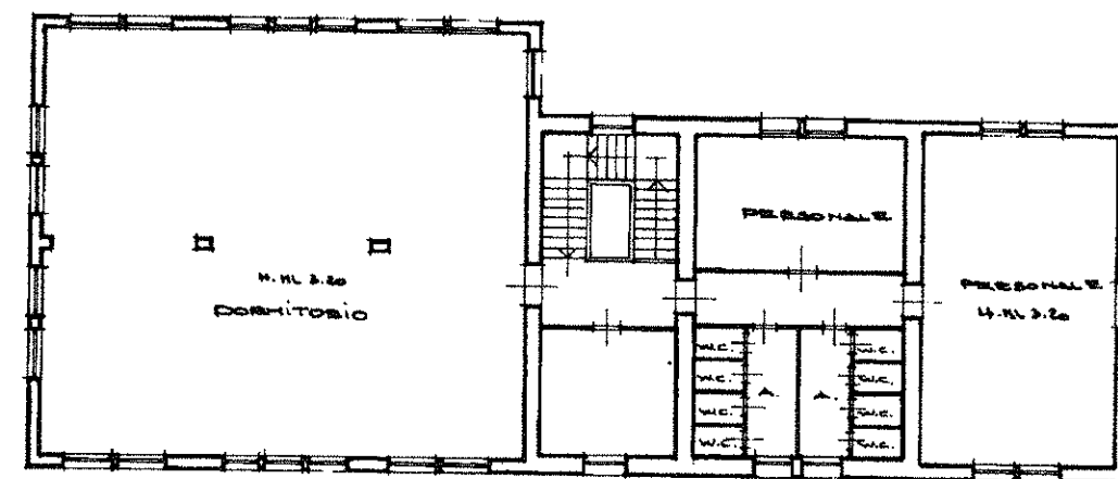
-PIANO TERZO-
